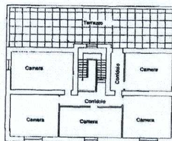
PIANTA PIANO PRIMO (h. = 3.32)
